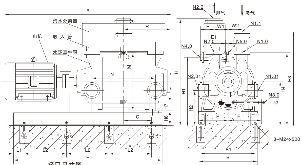
2BEX 303-353电机直联安装外形尺寸图
