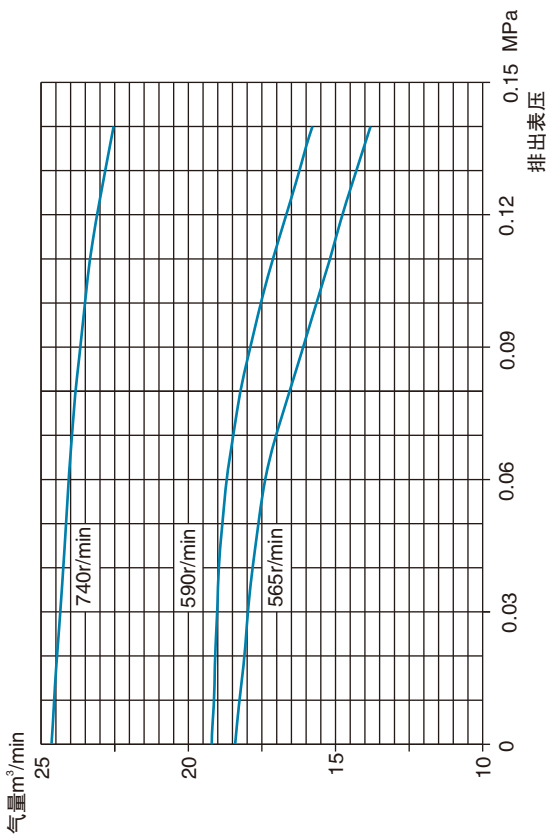
2BEX252-8 水环压缩机吸气量、轴功率曲线
