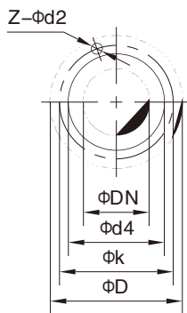
接口尺寸图
