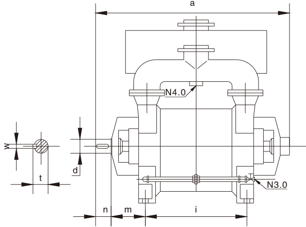
泵外形及安装尺寸
