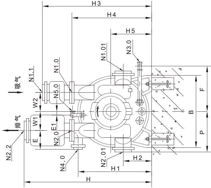
2BEX 503/505/603/605减速机传动安装外形尺寸图
